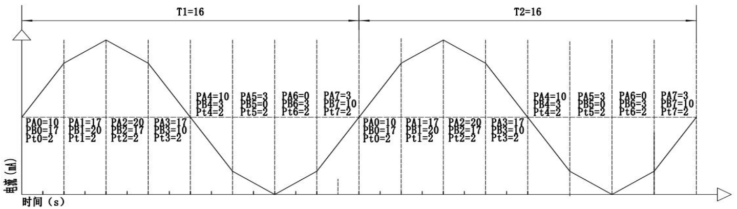
图 4.4 线编程输出近似正弦波
