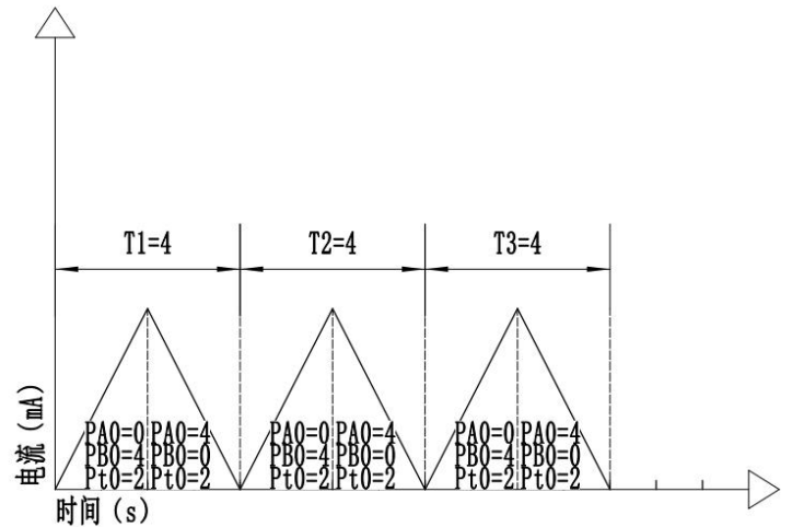
图 4.3 线编程输出三角波
