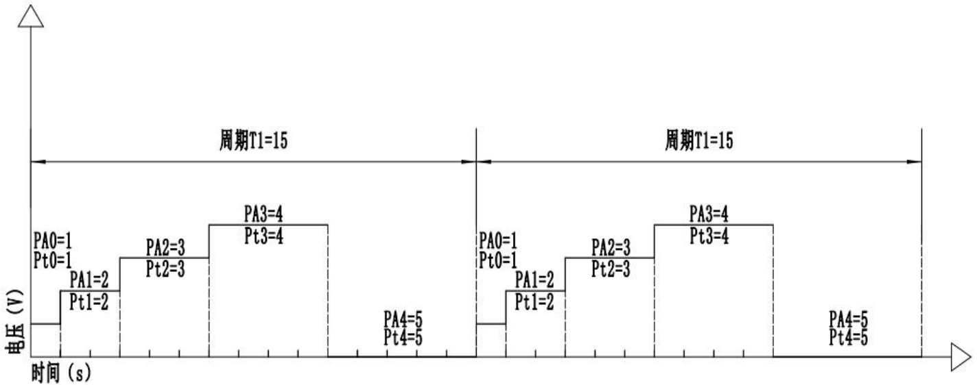
图 4.1 点编程输出多段方波曲线
