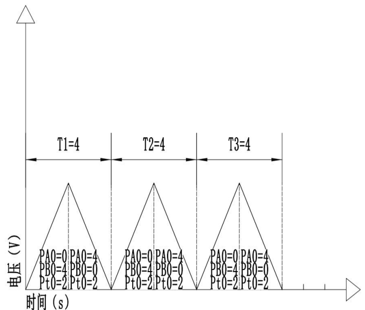
图 4.3 线编程输出三角波
