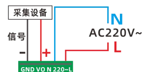
【交流版】模拟信号接线示意图
