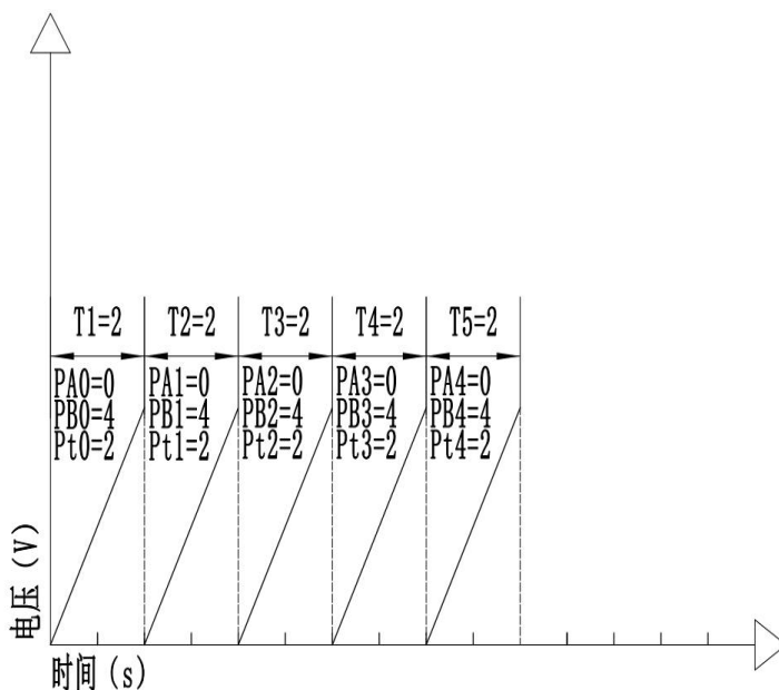
图 4.2 线编程输出锯齿波
