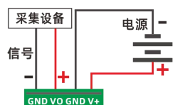
【直流版】模拟信号接线示意图
